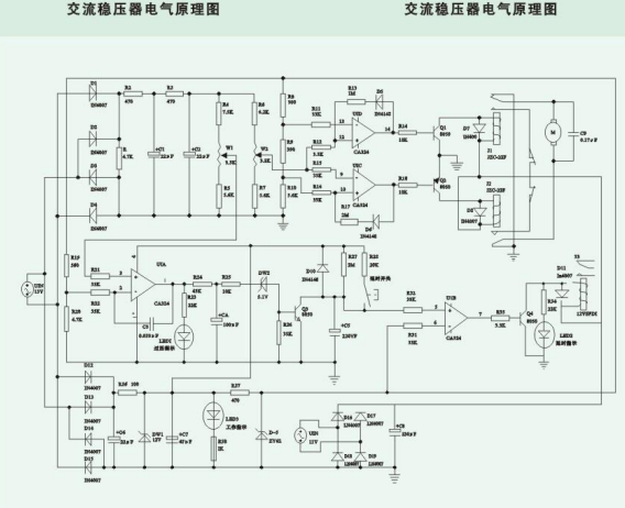
图6 三相5KVA-40KVA控制线路图仅供参考,如有改动,恕不另行通知
