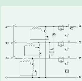
图5 补偿式三相高精度全自动交流稳压电器原理图
