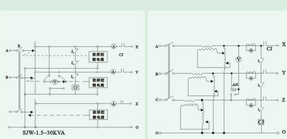
图4 SJW-1.5-30KVA三相高精度全自动交流稳压电器原理图
